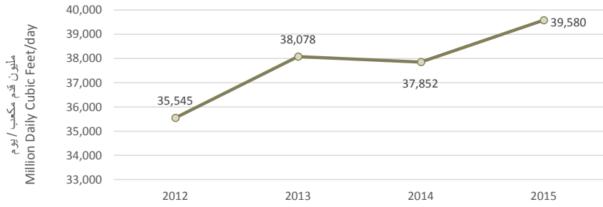
شكل 34: إنتاج الغاز المسوق في مجلس التعاون 2012-2015م Figure 34: Gas Production in GCC 2012-2016
