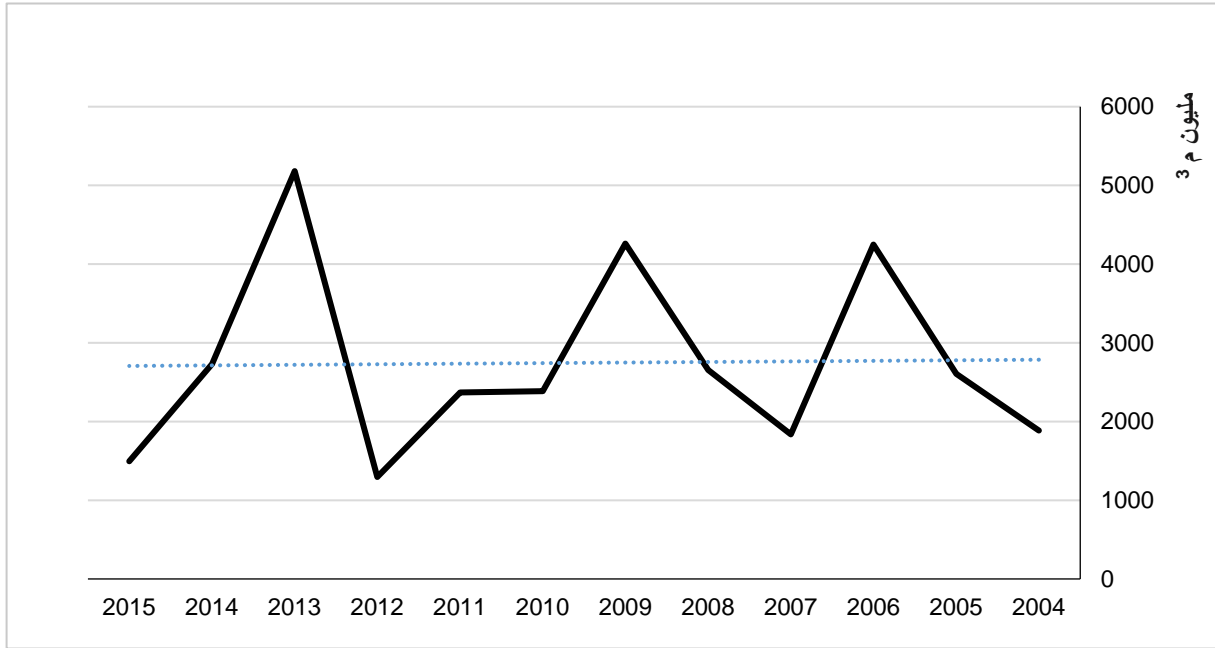
شكل 10: إجمالي كمية هطول الأمطار في دولة الإمارات العربية المتحدة خلال الفترة
