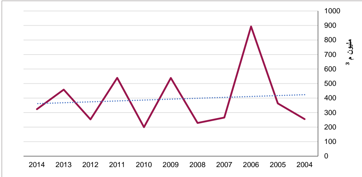
شكل 58: إجمالي كمية هطول الأمطار في دولة قطر خلال الفترة 2004-2014م
