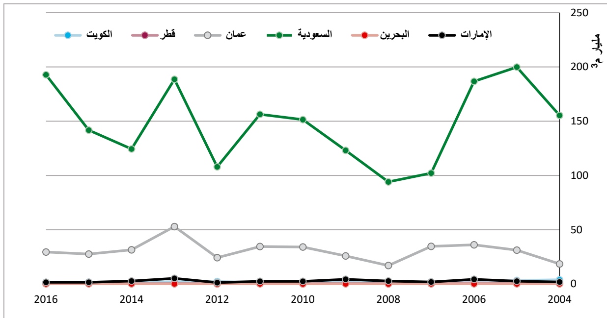
شكل 76: كميات هطول الأمطار في دول مجلس التعاون خلال الفترة 2004-2016م
