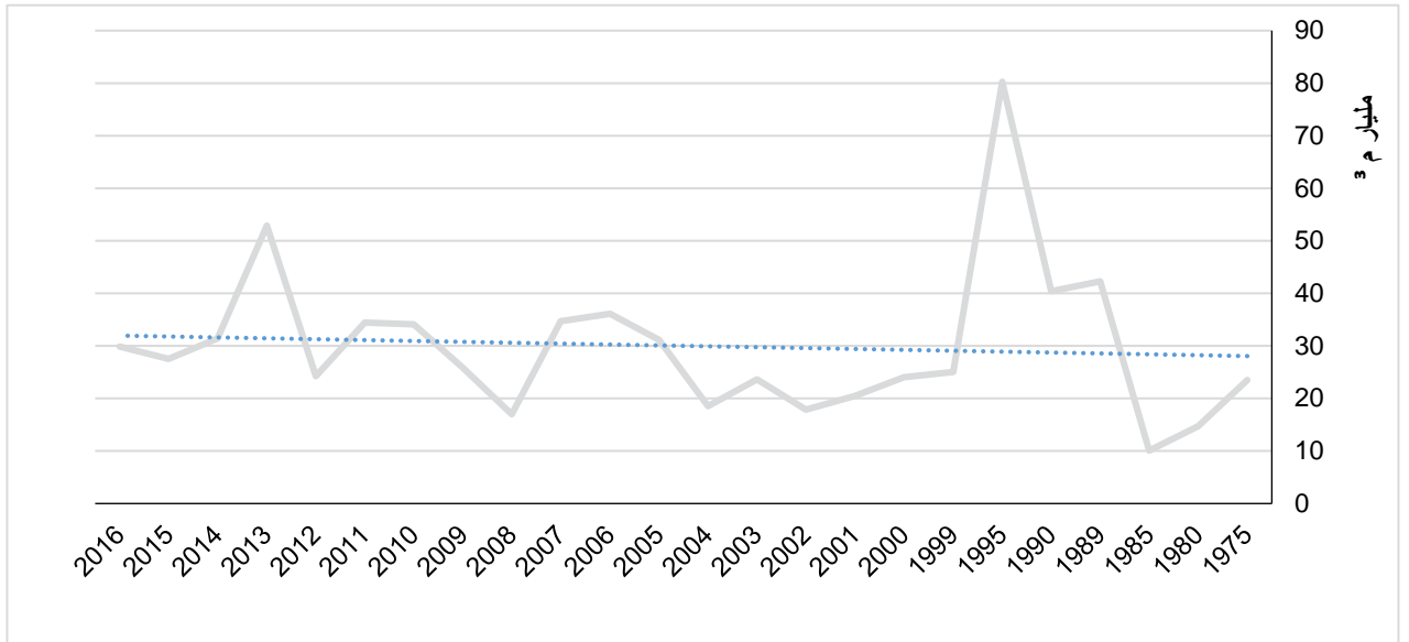
شكل 46: إجمالي كمية هطول الأمطار في سلطنة عمان خلال الفترة 1975-2016م
