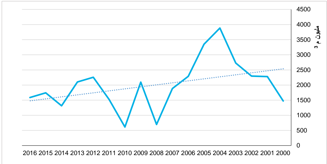
شكل 67: إجمالي كمية هطول الأمطار في دولة الكويت خلال الفترة 2000-2016م
