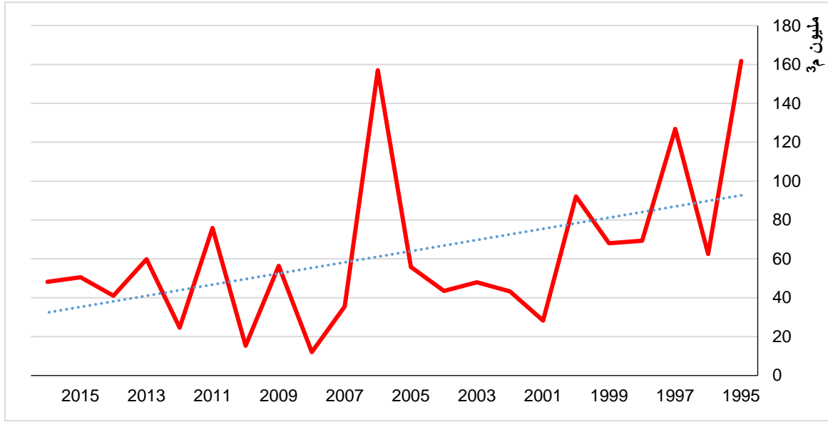
شكل 22: إجمالي كمية هطول الأمطار في مملكة البحرين خلال الفترة 1995-2016م
