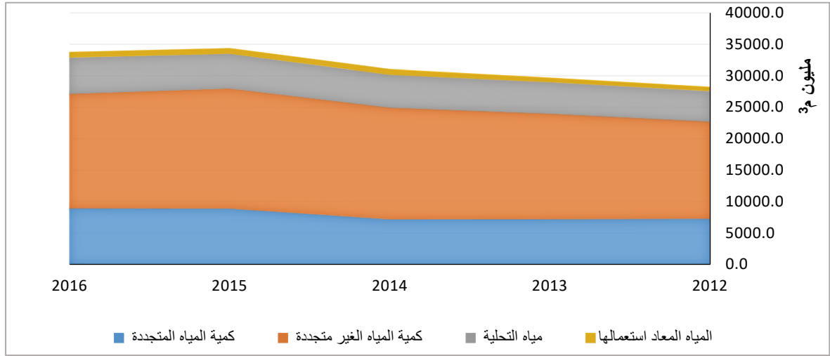
شكل 1: إجمالي كمية هطول الأمطار على مستوى دول مجلس التعاون خلال الفترة 2012-2016
