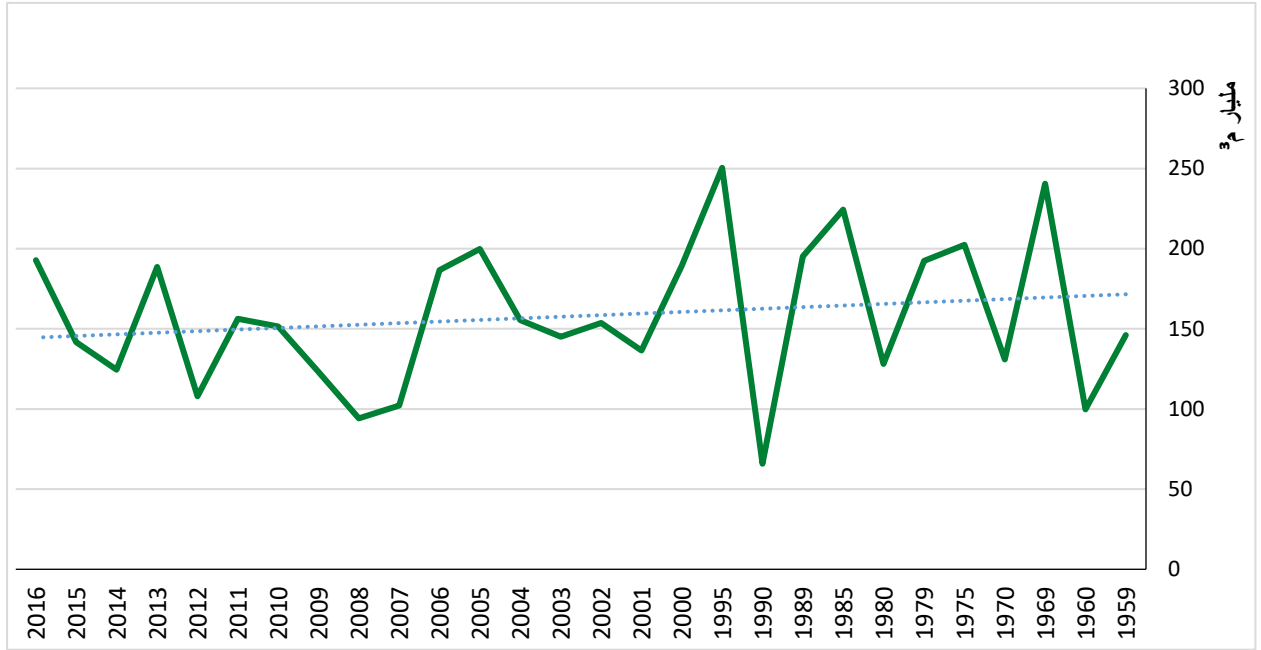
شكل 34: إجمالي كمية هطول الأمطار في المملكة العربية السعودية خلال الفترة 1959-2016م
